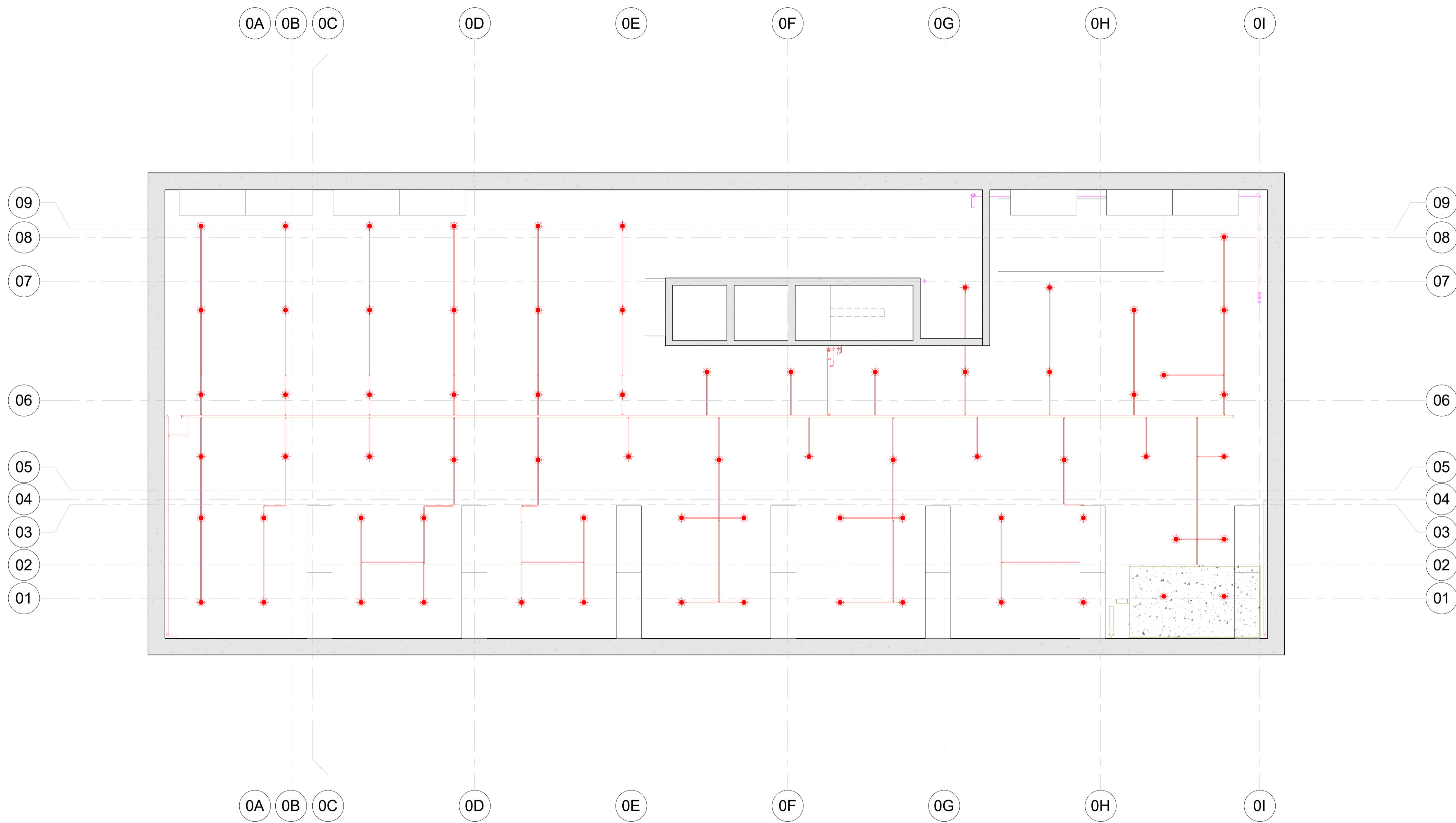
1 01-ERCP-Basement 2 1 : 100
