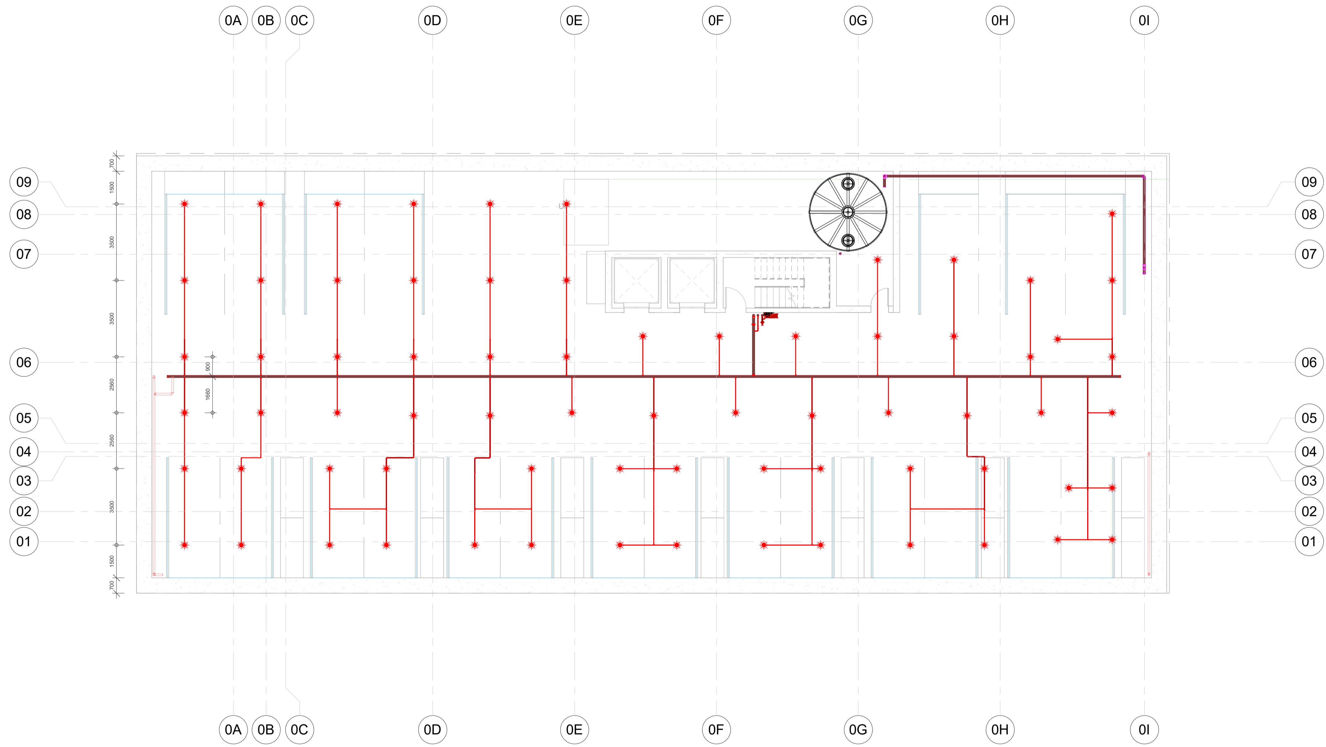
1 01-EM-Basement 2 1 : 100
